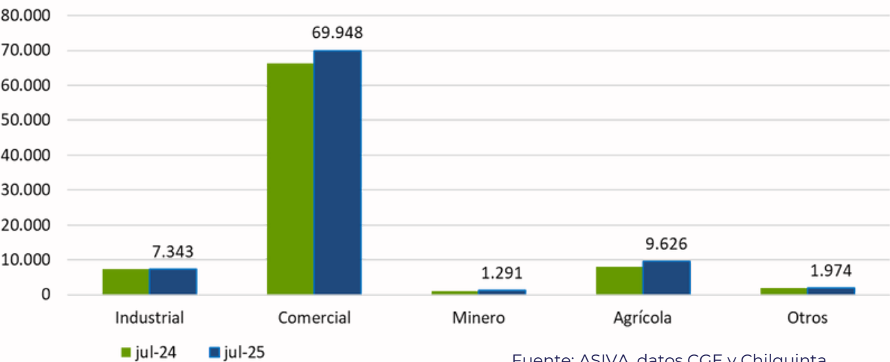
Venta de Energía Eléctrica (MWh)
