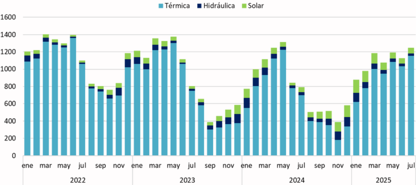
Generación de Energía Eléctrica (MWh)
